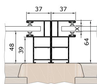
Kämpfer mit 2x Führungs- schiene KD37R / *GD37R
