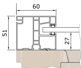
Führungsschiene K60AE / * G60AE
