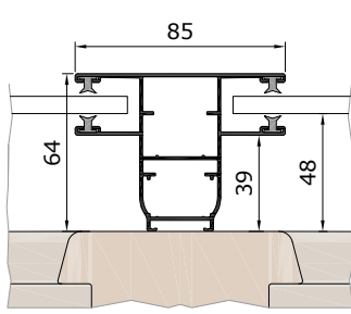
Doppel-Führungsschiene KD85R / *GD85R
