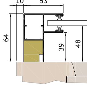
Führungsschiene KD53RT / *GD53RT
