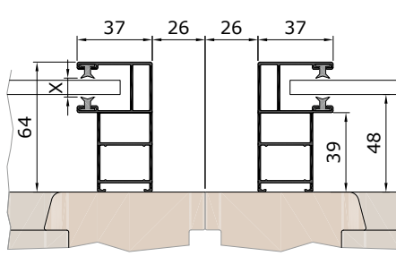
2x Führungsschiene mit KD37R / *GD37R
