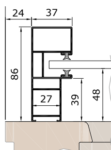
Führungsschiene KD37K / * GD37K
